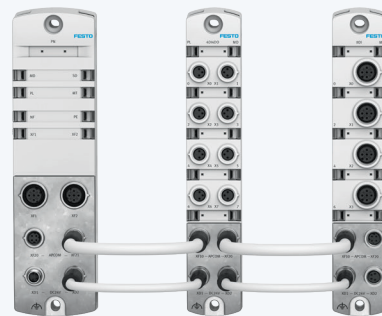
Decentralized remote I/O modules CPX-AP-I
